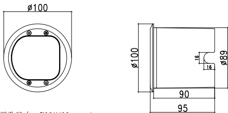
开孔尺寸: Ø90*H93mm ±1mm
